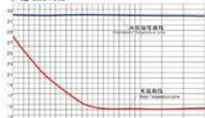
单池 SING POND
