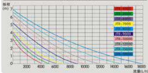
变频水泵曲线图
