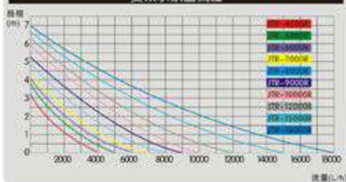
变频水泵曲线图
